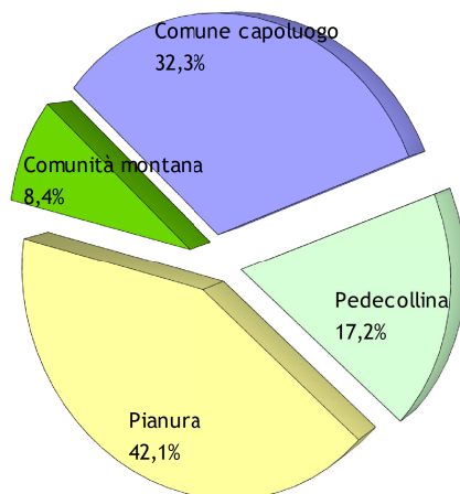
Popolazione per zone altimetriche
